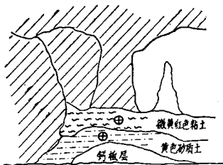
盘龙洞剖面(二)
