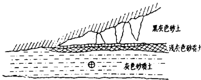
盘龙洞剖面(一)
