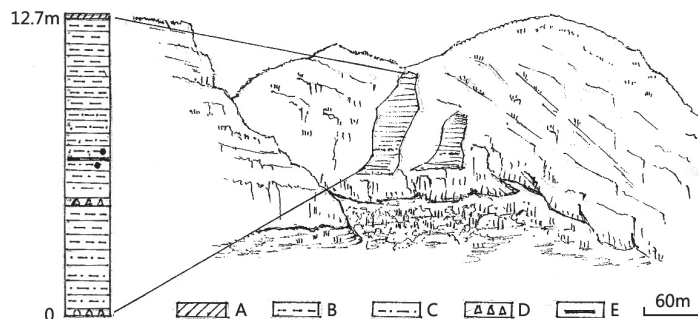
图 2 凤凰山地点地层剖面图
