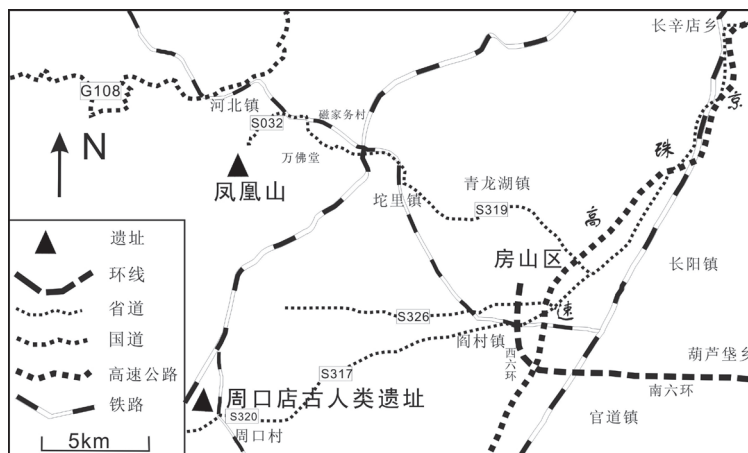
图 1 凤凰山地点地理位置图
