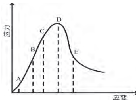
图 1 理想状态下岩石应力与应变关系曲线
