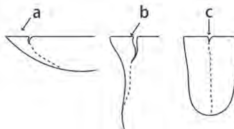
图 3 破裂类型: a 弯曲破裂; b 赫兹破裂; c 楔作用破裂 (据 Odell, 2004) [15]
