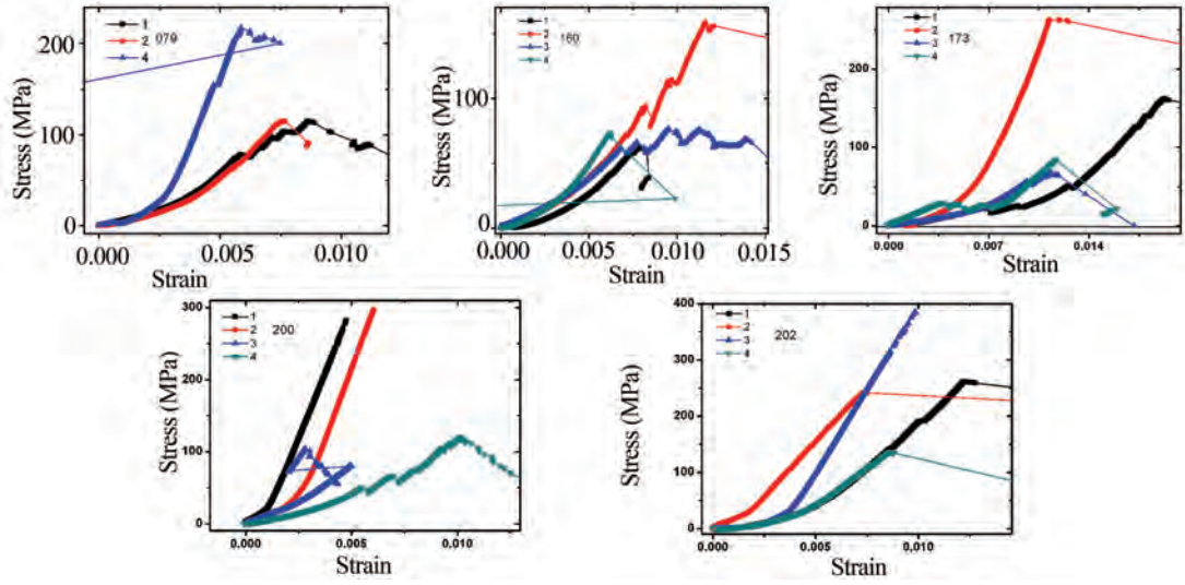
图 4 水洞沟遗址石料应力 - 应变曲线
