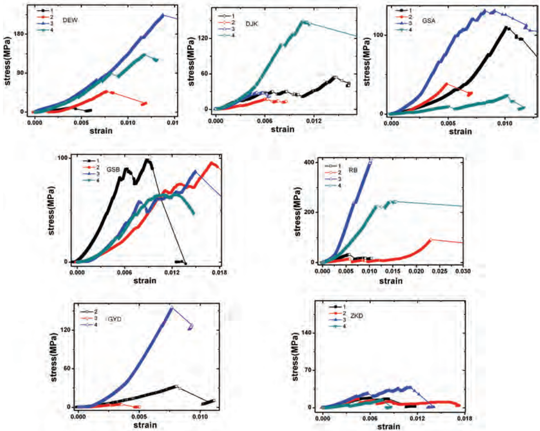
图 5 不同石料应力 - 应变曲线
